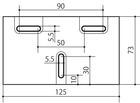
取付面拡大図（単位：mm）
