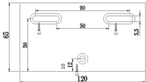
取付板拡大図 (単位: mm)
